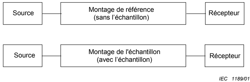
Figure A.1b – Technique du montage de référence
