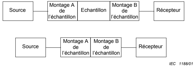
Figure A.1a – Technique d'insertion
